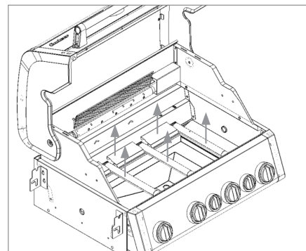
Stap 3: Verwijder de branderbuizen en vlambruggen verwijderen.
